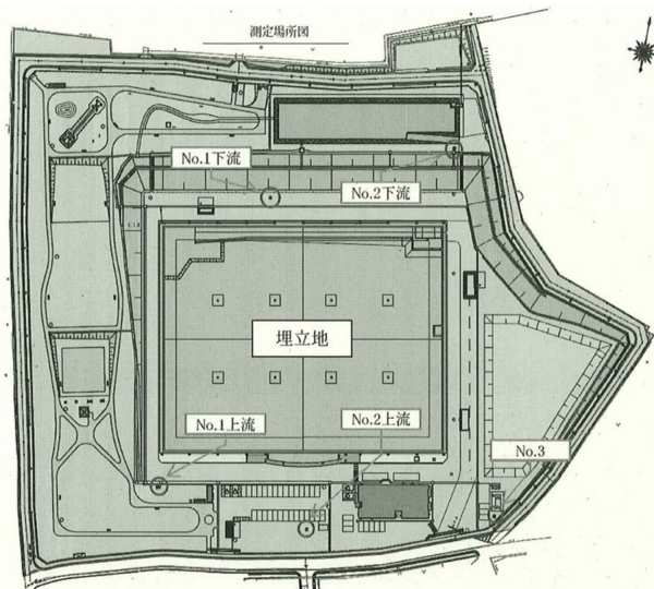
図1 測定場所図
