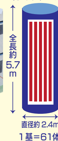
乾式キャスク
